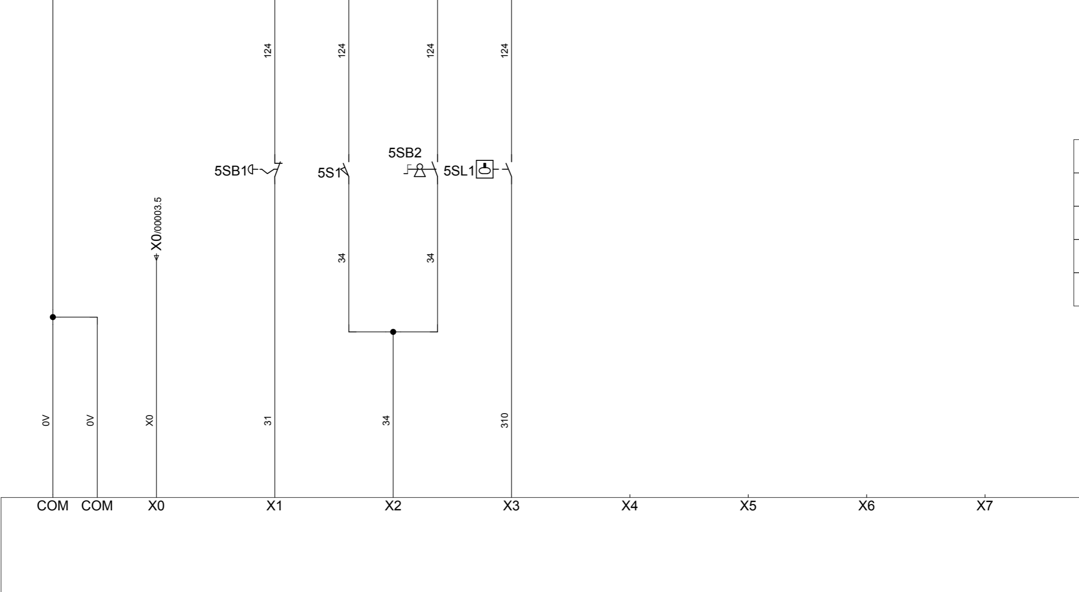
CONN.B
